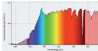
Klarer Himmel morgens nach Sonnenaufgang Ri SW
